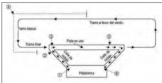
Figura 1. Posiciones designadas de las aeronaves desde un punto de vista de la torre de control del aeródromo (véase 6.6.2)
