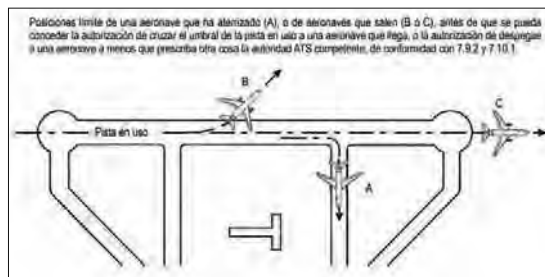
Figura 3. Separación entre aeronaves que llegan y salen (véanse 6.9.2 y 6.10.1)
